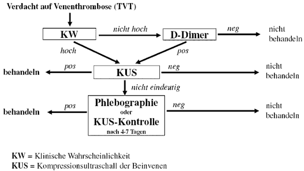
Abbildung 1: Diagnostischer Algorithmus bei Verdacht auf Venenthrombose
