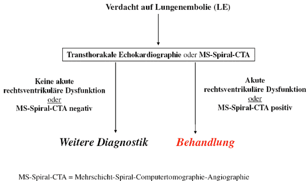
Abbildung 2: Diagnostischer Algorithmus bei Verdacht auf Lungenembolie mit hohem klinischen Risiko (instabiler Patient)
